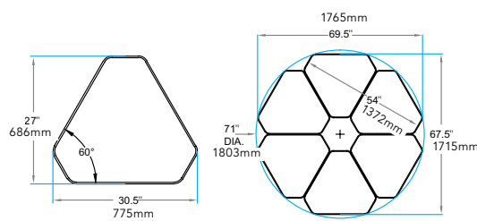
Model 04505. Interchange Mini Diamond Student Desk
